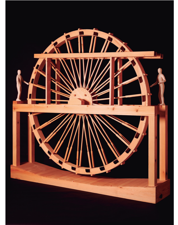
Rota para el achique minero de las minas de Riotinto (Huelva)
