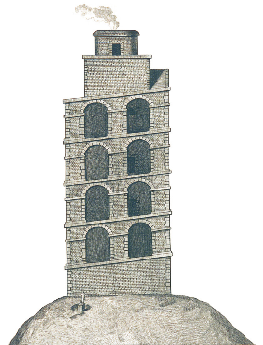
Alzado de la Torre de Hércules. En: José Cornide. Investigaciones sobre la fundación y fábrica de la torre llamada de Hércules 1792. Copyright © Patrimonio Nacional
